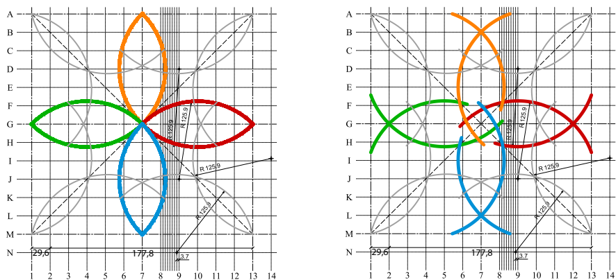
Abb. 1 Gewölbe über der Reiterstiege, Hradschin Prag, um 1502. Dekonstruktion in der Grundrissfiguration
